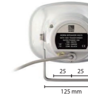
Mål - Monteringsbøjle
